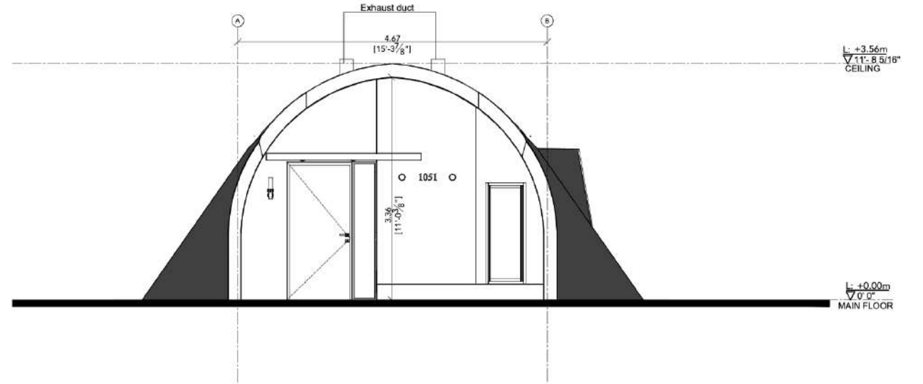
SCALE = 1:50 1 A4 ELEVATION 1
