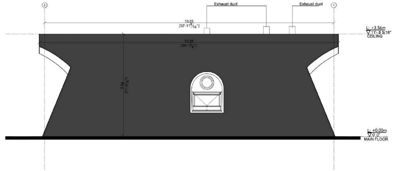
SCALE = 1:50 2 A4 ELEVATION 2
