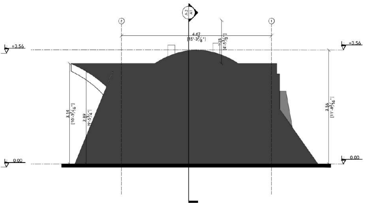
SCALE = 1:50 4 A2 ELEVATION 4
