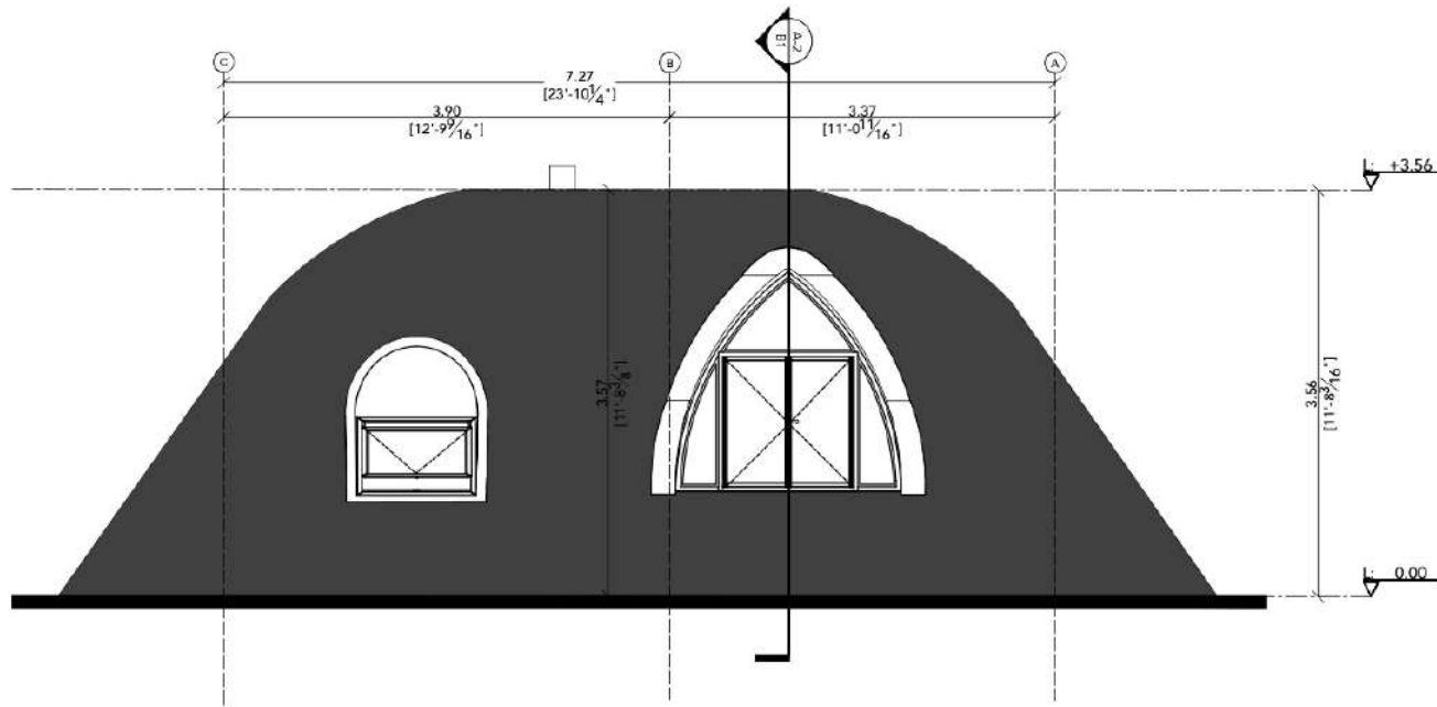
SCALE = 1:50 3 A2 ELEVATION 3
